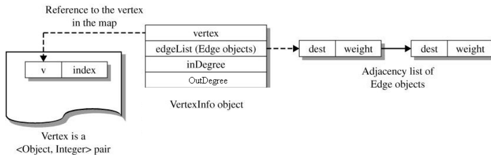
Gambar 29.13 Cara penyimpanan vertex dalam object VertexInfo
