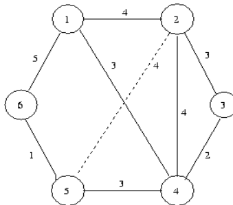
Gambar 29.8 Graph tak berarah dengan pembobot
