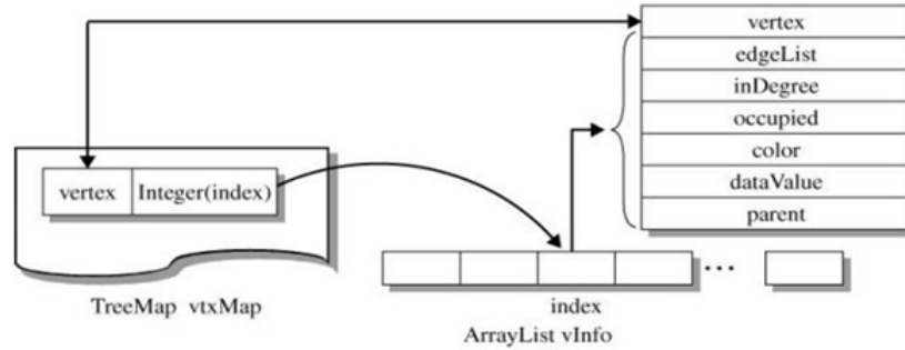
Gambar 29.14 Keterkaitan HashMap vtxMap dan ArrayList vInfo
