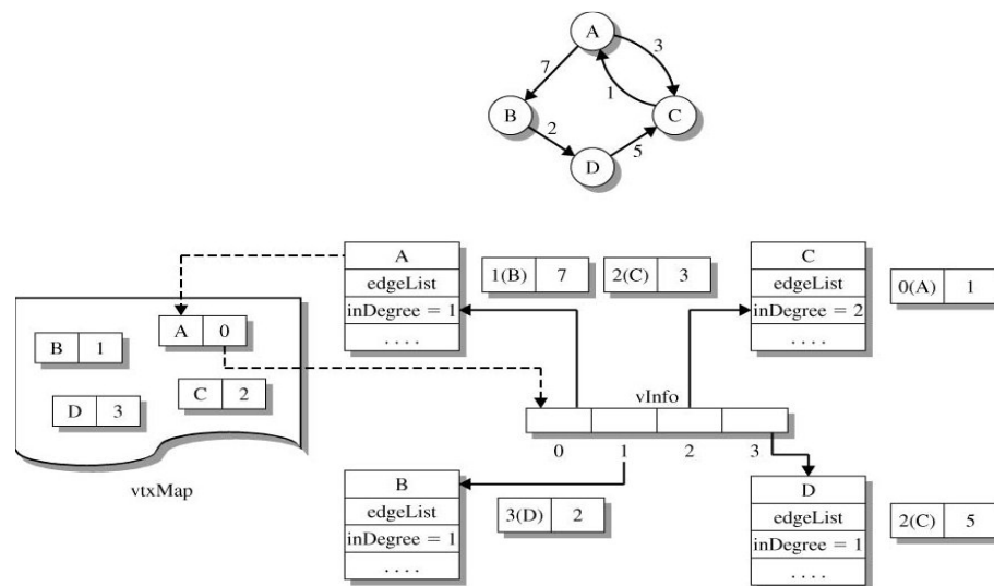
Gambar 29.15 Graph, beserta data yang tersimpan di vtxMap dan ArrayList vInfo.
