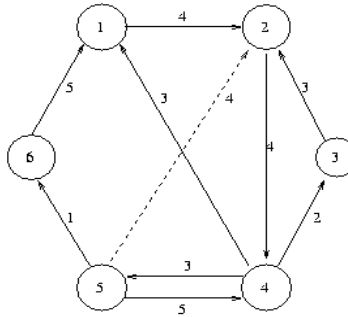
Gambar 29.7 Graph berarah dengan pembobot
