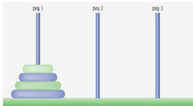
Gambar 1. Menara Hanoi
