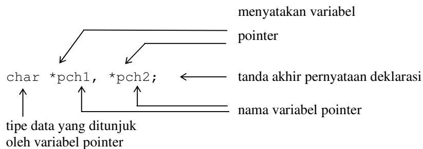
Gambar 1.3 Ilustrasi pendeklarasian variabel pointer
