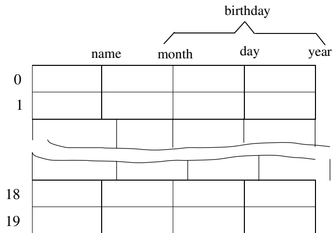
Gambar 1.4 Array dari struktur
