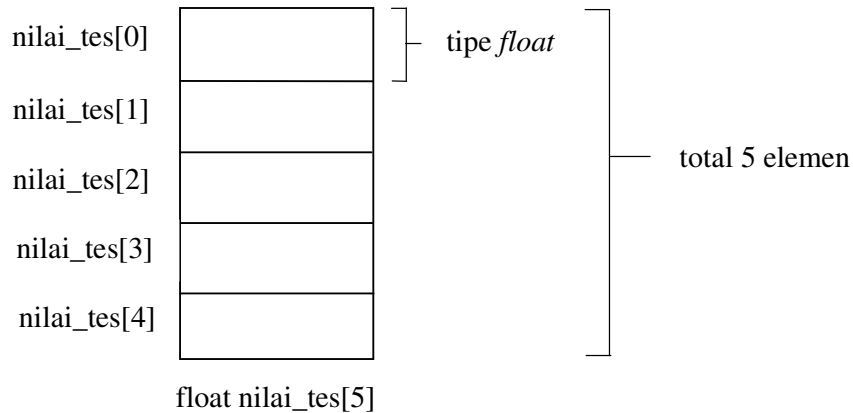
Gambar 1.1 Array berdimensi satu
