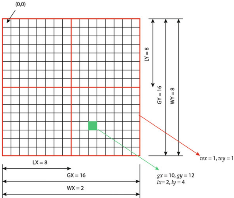
Fig. 5.10 NDRange
