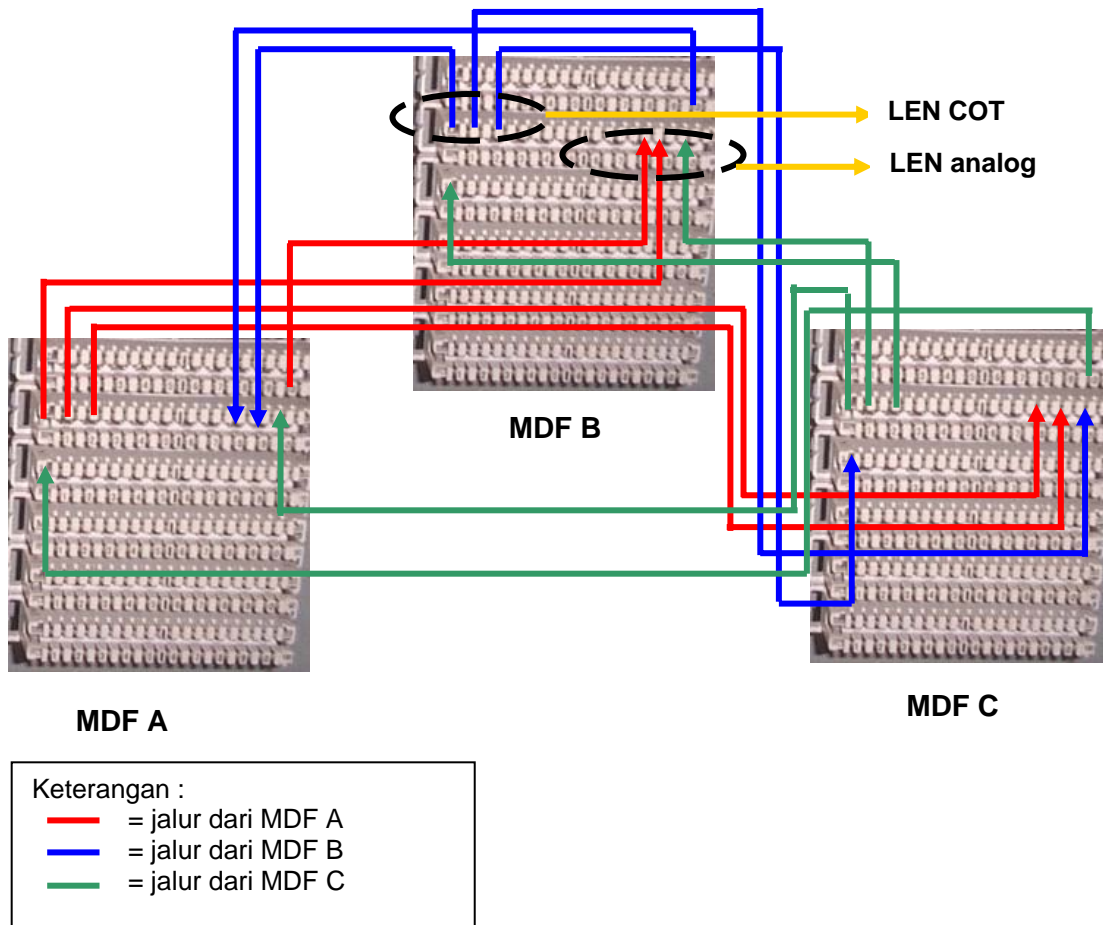
Gambar 9.2. Per kabelan antar MDF di PABX
