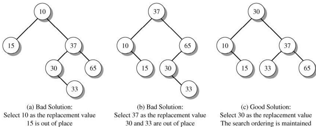
Gambar 2. Mencari Pengganti dengan Nilai yang Tepat
