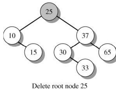
Gambar 1. Menghapus Node Root 25
