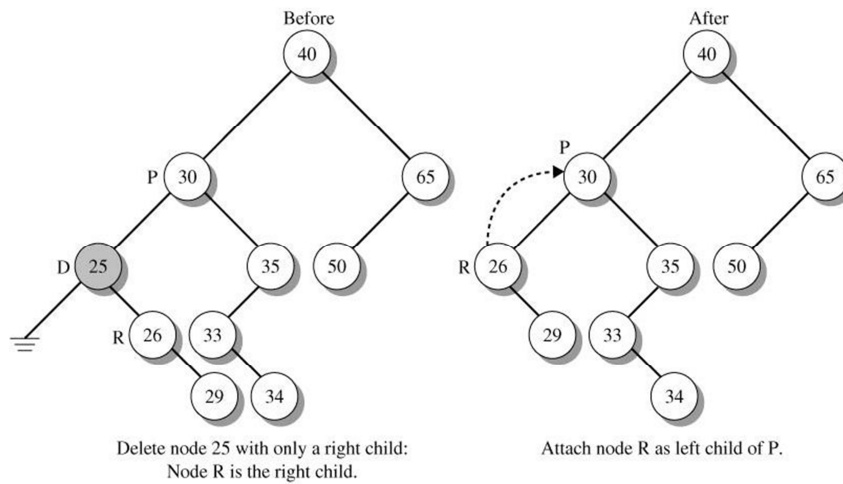
Gambar 4. Contoh 2, menghapus node yang memiliki 1 anak
